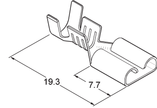
Düz Tip / Straight Type
