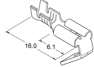
Erkek-Dişi Düz Tip Piggyback Straight Type
