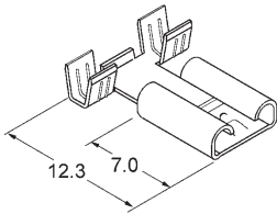
Tırnaklı Bayrak Tip / Snap-in Flag Type
