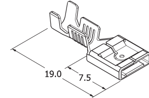
Düşük Takma Kuvvetli Low Insertion Force (LIF)
