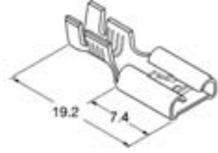
Tırnaklı Düz Tip / Snap-in Receptacle
