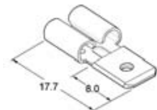
Erkek-Dişi Düz Tip / Piggyback Straight Type
